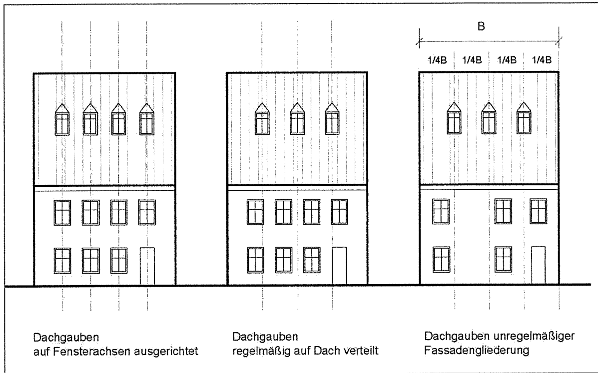
Abbildung 4: Dachgauben
