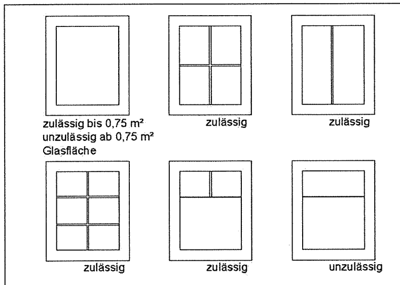
Abbildung 6: Fenstergliederung Sprossen
